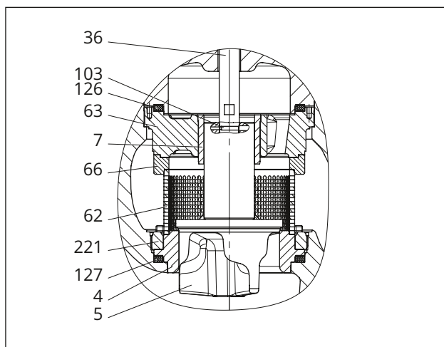
Bild 9: Ventil Typ 251GR · Varianten der Garniturausführung · geschraubter Sitz und Kegel mit Strömungsteiler ST1
