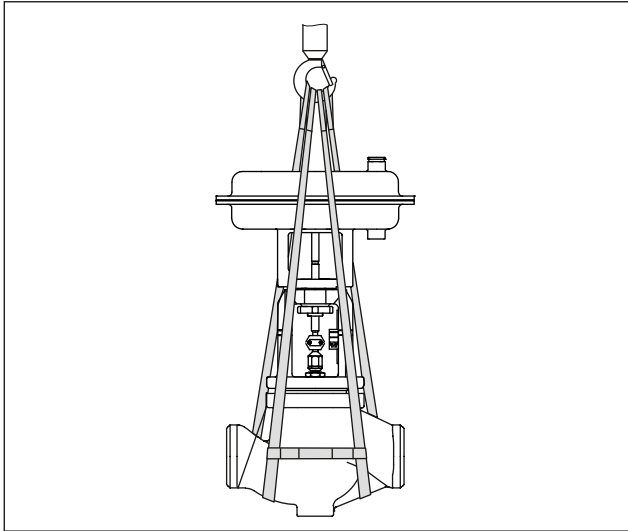
Bild 19: Heben eines Stellventils mit Anschweißenden (Beispieldarstellung): Die angeschlagenen Hebeschlingen sind untereinander mit einem Verbinderring gegen Abrutschen gesichert.
