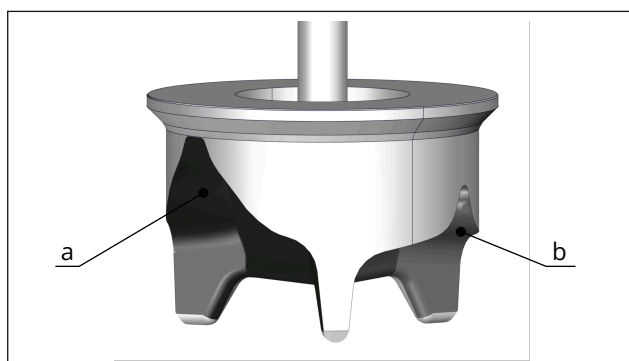
Bild 28: V-Port-Kegel (Beispieldarstellung)
