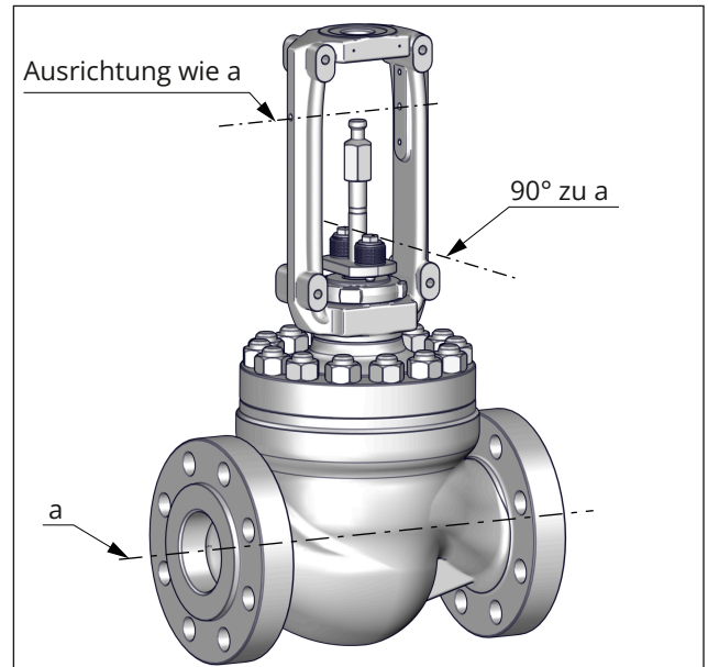
Bild 35: Ausrichtung der Packungsbrille im Joch
