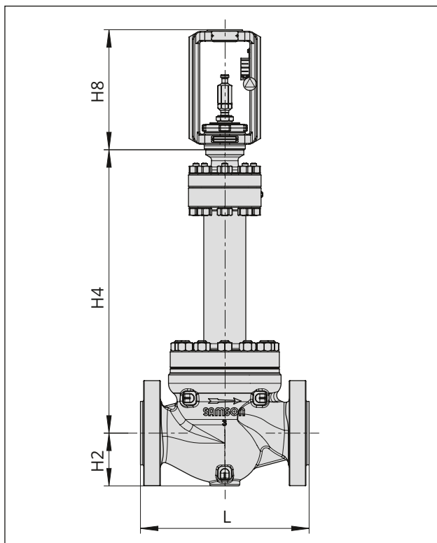
Bild 16: Ventil Typ 251GR in Ausführung mit Balgteildichtung
